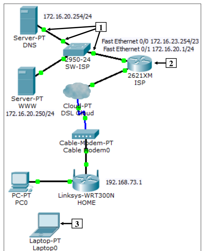
Figura 10(a) - Rede de computadores
